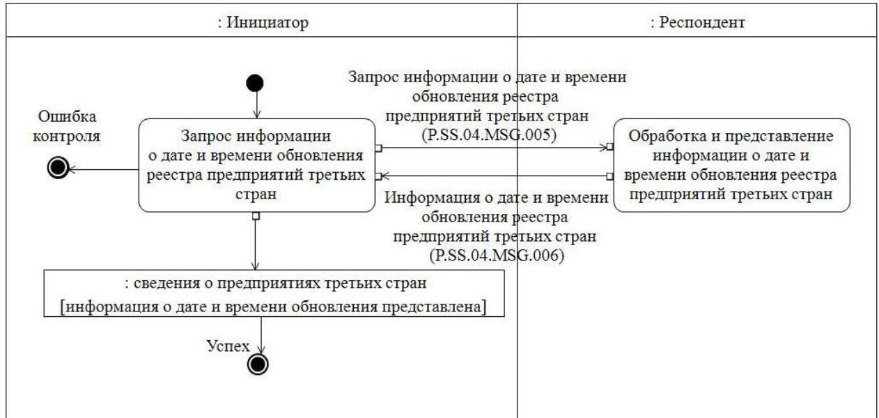
Рис. 7. Схема выполнения транзакции общего процесса «Получение информации о дате и времени обновления реестра предприятий третьих стран» (P.SS.04.TRN.004)
