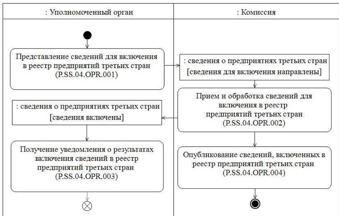
Рис. 5. Схема выполнения процедуры «Включение сведений в реестр предприятий третьих стран» (P.SS.04.PRC.001)
