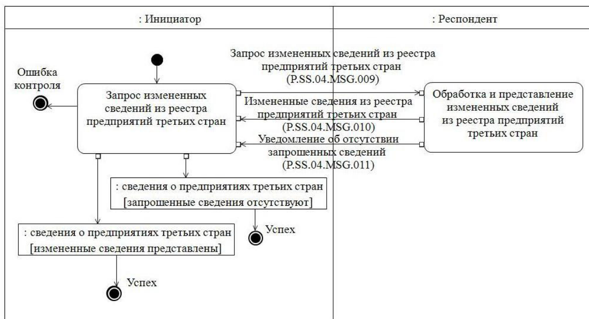
Рис. 9. Схема выполнения транзакции общего процесса «Получение измененных сведений из реестра предприятий третьих стран» (P.SS.04.TRN.006)
