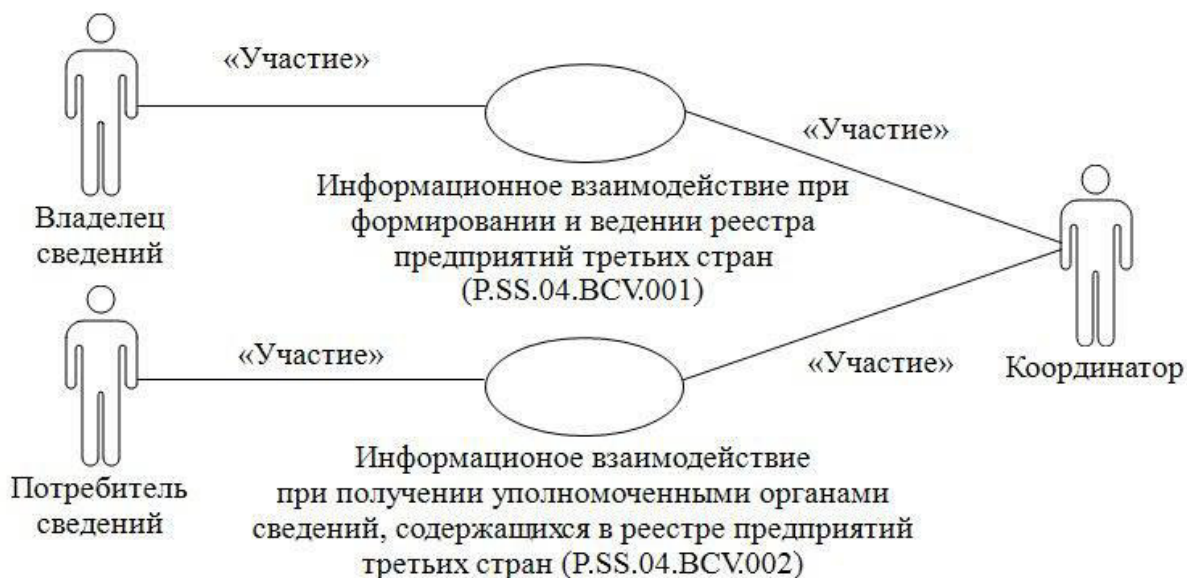
Рис. 1. Структура информационного взаимодействия между уполномоченными органами и Комиссией
