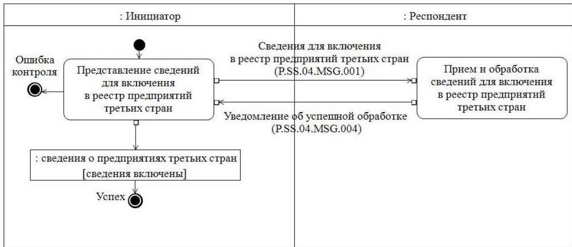
Рис. 4. Схема выполнения транзакции общего процесса «Передача сведений для включения в реестр предприятий третьих стран» (P.SS.04.TRN.001)
