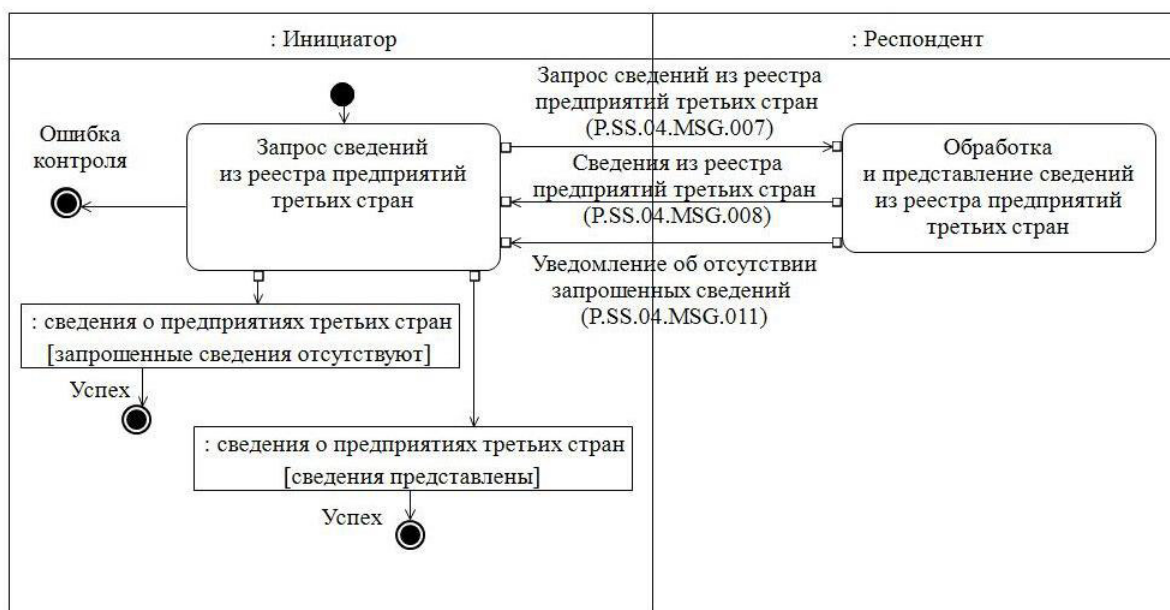
Рис. 8. Схема выполнения транзакции общего процесса «Получение сведений из реестра предприятий третьих стран» (P.SS.04.TRN.005)
