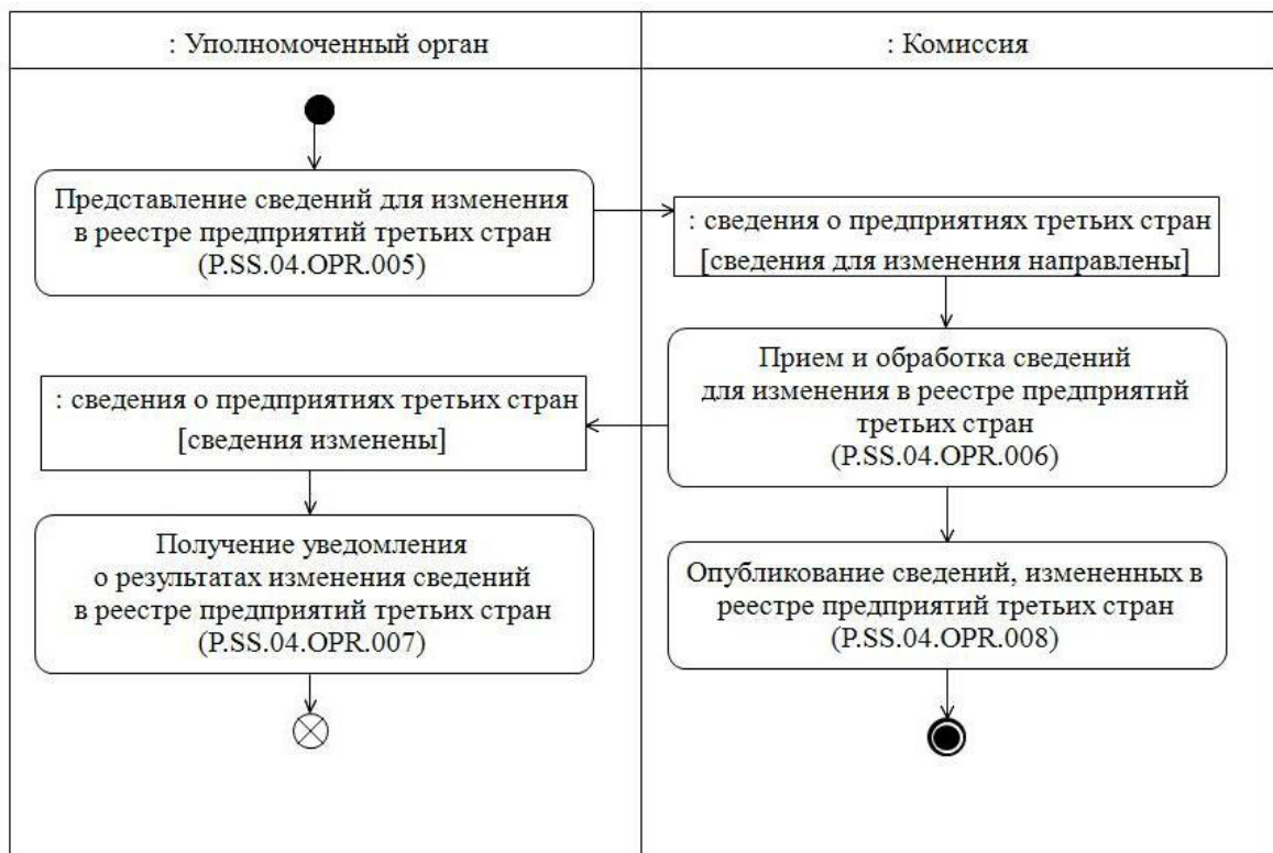
Рис. 6. Схема выполнения процедуры «Изменение сведений в реестре предприятий третьих стран» (P.SS.04.PRC.002)
