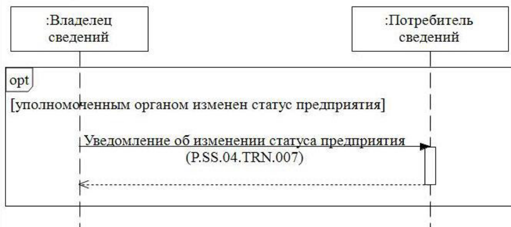
Рис. 2. Схема выполнения транзакций общего процесса при уведомлении уполномоченных органов об изменении статуса предприятия, включенного в реестр предприятий третьих стран
