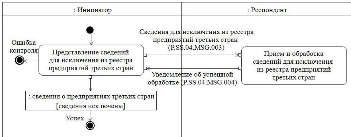
Рис. 6. Схема выполнения транзакции общего процесса «Передача сведений для исключения из реестра предприятий третьих стран» (P.SS.04.TRN.003)
