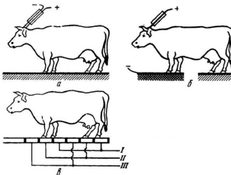
Рис. 2.5. Способы обездвиживания крупного рогатого скота: а) одно контактный; б) двух контактный; в) к пластинам пола
