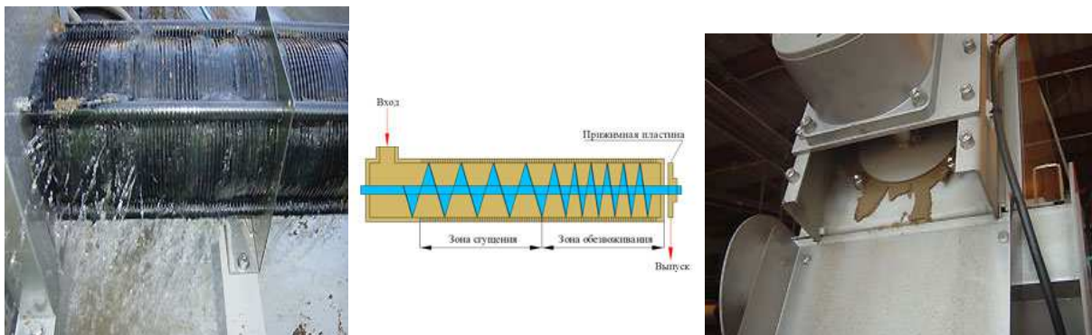
Рис. 2.85 Шнековый дегидратор (конструкция).
