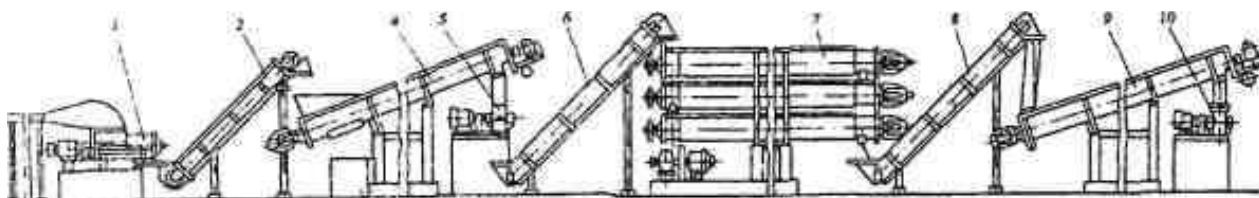
Рис. 2.68 Схема линии К7-ФКЕ производства сухих кормов животного происхождения: 1 - измельчитель; 2 - элеватор; 3 - жироловка; 4 - обезвоживатель; 5, 10 - дробилки; 6, 8 - элеваторы обогреваемые; 7 - сушильный агрегат; 9 - охладитель
