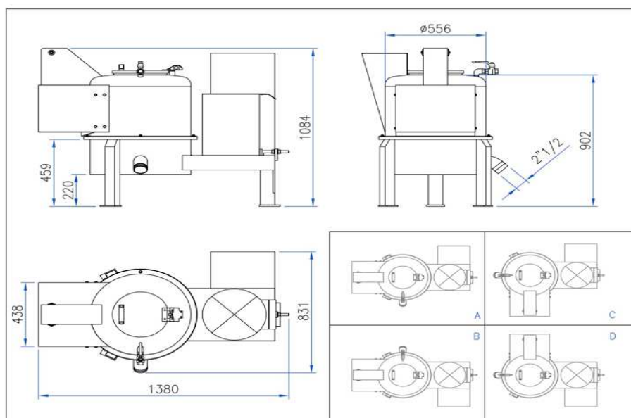
Рис. 2.166. Центрифуга
