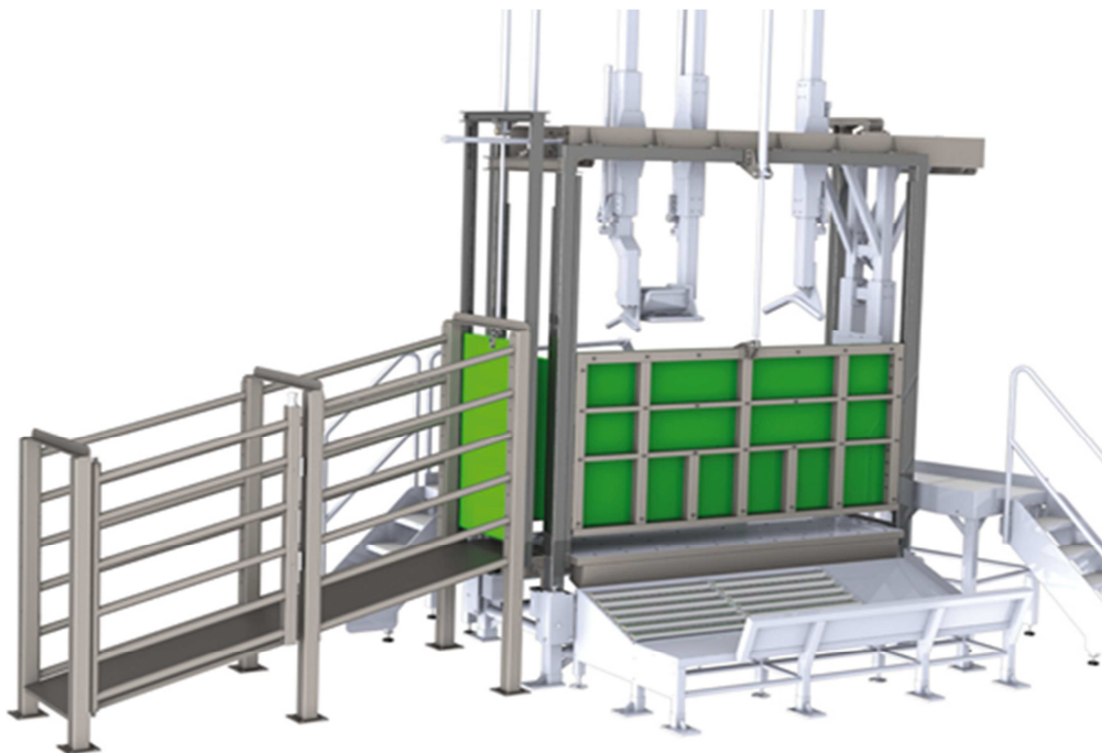
Рис. 2.94 Бокс оглушения КРС и телят мощностью от 100 голов/час
