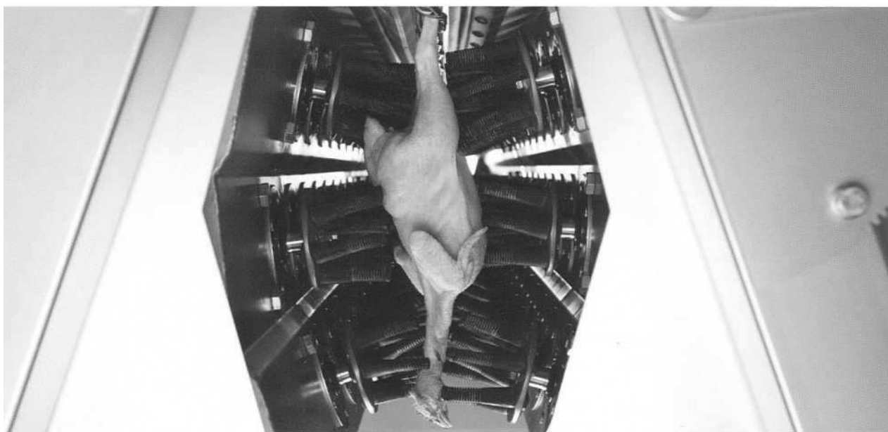
Рис. 2.38 Обработка птицы в аппарате для удаления пера
