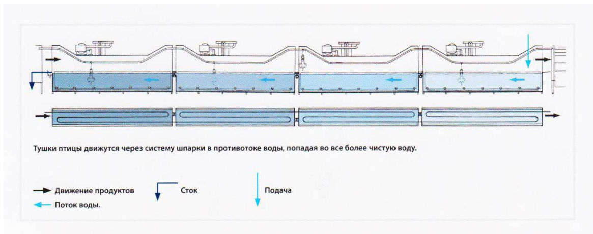
Рис. 2.37 Направления движения продуктов и воды при шпарке в воде
