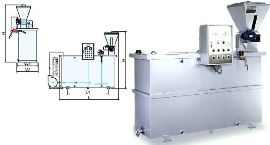
Рис. 2.79 Полимерная станция
