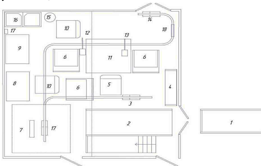
Рис. 2.180 Схема размещения и состав основного оборудования
