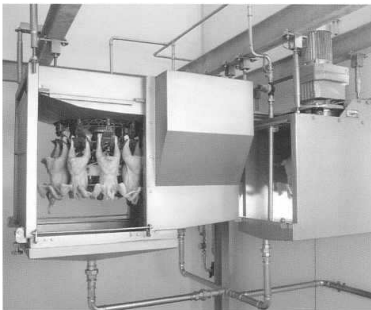
Рис. 2.43 Камеры охлаждения на поворотных колесах
