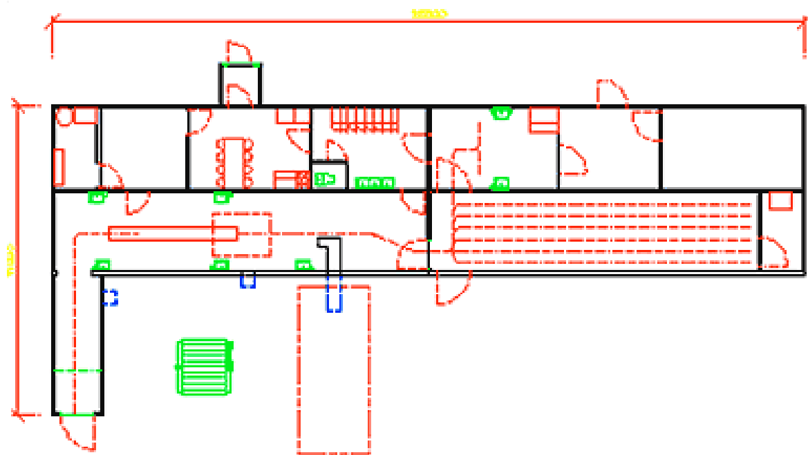
Рис. 2.19 Принципиальная схема бойни для оленей и мелкого рогатого скота
