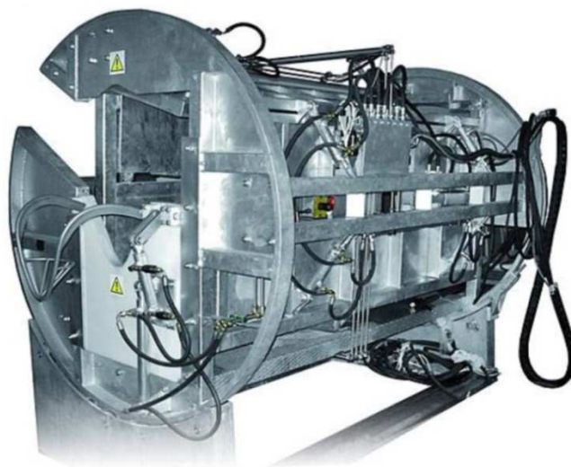
Рис. 2.193 Бокс для халяльного убоя КРС
