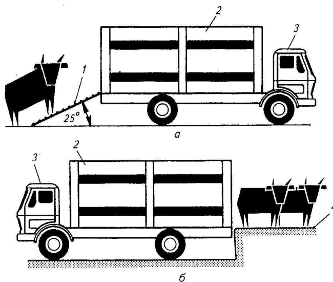
Рис. 2.1. Схема загрузки крупного рогатого скота в скотовозы: а – по трапу; б – с эстакады-платформы: 1 – трап; 2 – кузов; 3 – автомобиль; 4 – эстакада платформы
